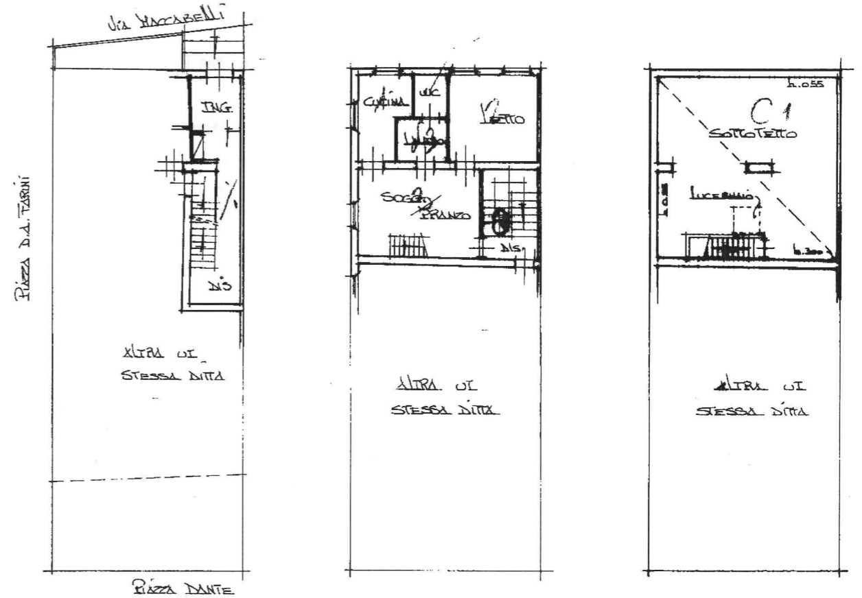
Pianta Piano Terra Pianta Piano Primo h. 300 Pianta Sottotetto
